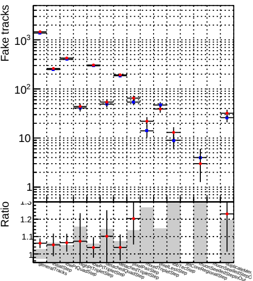
Number —●— DQM_mkFit_XiMinusPUold-lowpt
