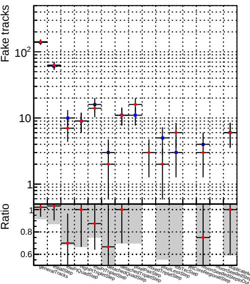
Number —●— DQM_mkFit_XiMinusPUold-lowpt
