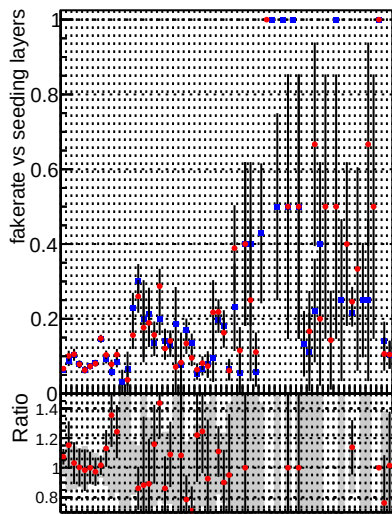
Fake rate vs. —•— DQM mkFit XiMinusPU_retrain2-lowpt —•— DQM mkFit XiMinusPUold-lowpt
