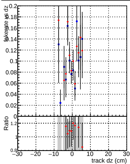
—•— DQM_mkFit_XiMinusPU_retrain2-lowpt —•— DQM_mkFit_XiMinusPUold-lowpt
