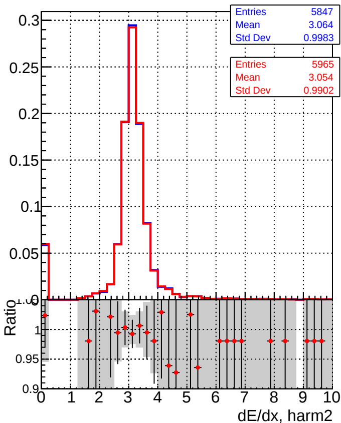
DQM_mkFit_XiMinusPU_retrain2-lowpt DQM_mkFit_XiMinusPUold-lowpt
