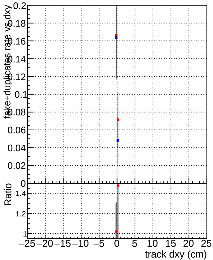
DQM_mkFit_XiMinusPU_retrain2-lowpt DQM_mkFit_XiMinusPUold-lowpt
