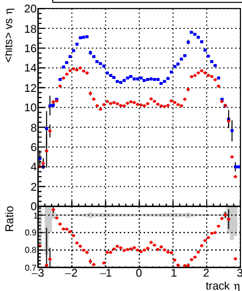
— DQM_mkFit_XiMinusPU_retrain2-lowpt — DQM_mkFit_XiMinusPUold-lowpt mean hits vs \eta
