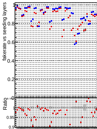
Fake rate vs. — DQM_mkFit_XiMinusPU_retrain2-lowpt — DQM_mkFit_XiMinusPUold-lowpt
