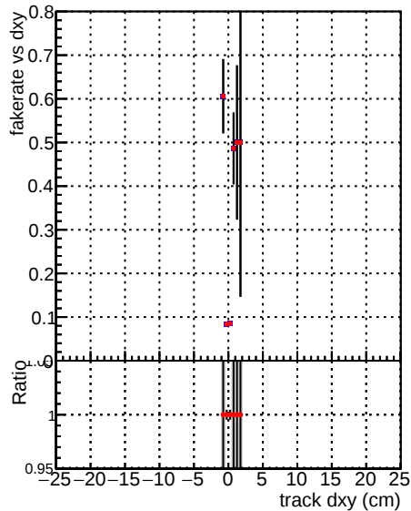
—●— DQM_mkFit_XiMinusPU_retrain2-lowpt —●— DQM_mkFit_XiMinusPUold-lowpt
