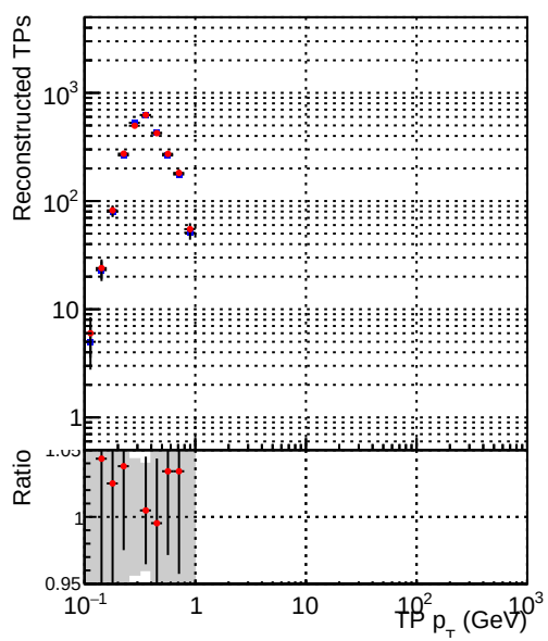
—•— DQM_mkFit_XiMinusPU_retrain2-lowpt —•— DQM_mkFit_XiMinusPUold-lowpt
