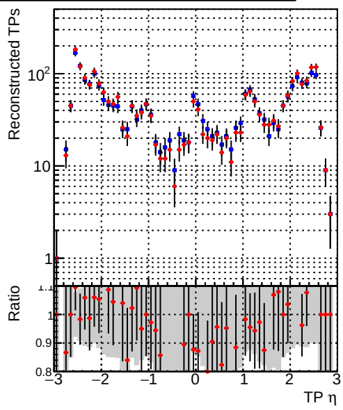
—•— DQM_mkFit_XiMinusPU_retrain2-lowpt —•— DQM_mkFit_XiMinusPUold-lowpt
