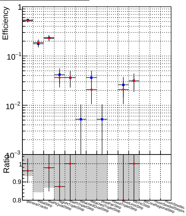
DQM_mkFit_XiMinusPU_retrain2-lowpt DQM_mkFit_XiMinusPUold-lowpt
