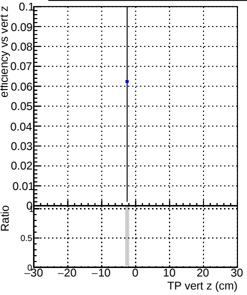
Efficiency vs TP vert z (cm) Legend: DQM_mkFit_XiMinusPU_retrain2-lowpt DQM_mkFit_XiMinusPUold-lowpt
