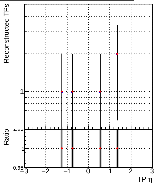
Legend: - \blacksquare DQM_mkFit_XiMinusPU_retrain2-lowpt - \bullet DQM_mkFit_XiMinusPUold-lowpt
