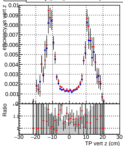
Efficiend —●— DQM_mkFit_XiMinusPUold-lowpt
