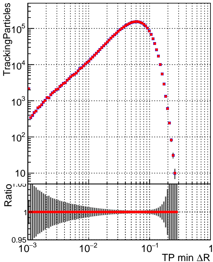
■ DQM_mkFit_XiMinusPU_retrain2-lowpt ● DQM_mkFit_XiMinusPUold-lowpt
