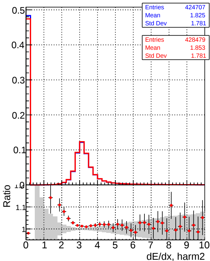
DQM_mkFit_XiMinusPU_retrain2-lowpt DQM_mkFit_XiMinusPUold-lowpt
