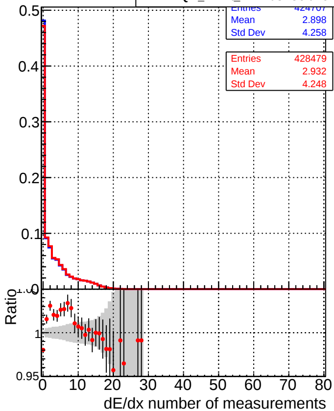
DQM_mkFit_XiMinusPU_retrain2-lowpt DQM_mkFit_XiMinusPUold-lowpt
