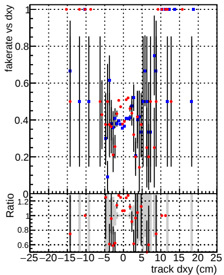
—◆— DQM_mkFit_XiMinusPU_retrain2-lowpt —◆— DQM_mkFit_XiMinusPUold-lowpt
