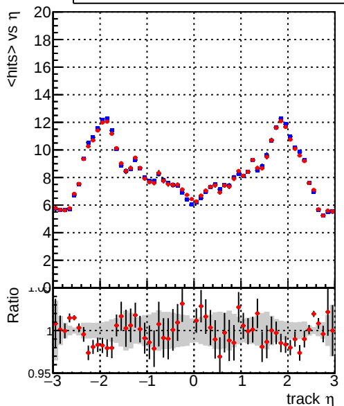
— DQM_mkFit_XiMinusPU_retrain2-lowpt — DQM_mkFit_XiMinusPUold-lowpt mean hits
