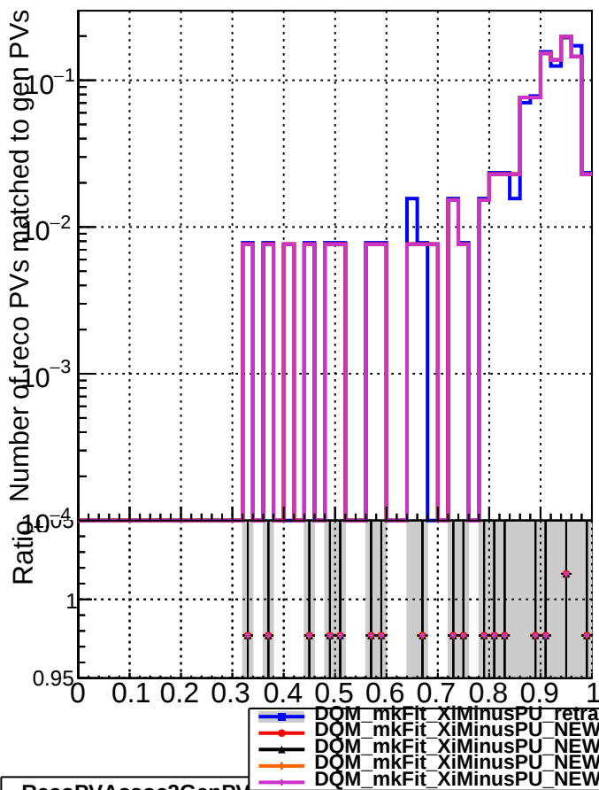
RecoPVAssoc2GenPVmatched_missing DQM_mkrfit
