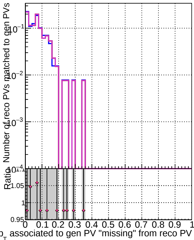
RecoPVAssoc2GenPVmatched_missing DQM_mkrfit
