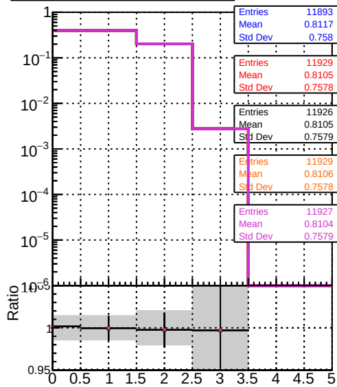
Legend: DQM mkFit XiMinusPU tetrain2-lowpt, DQM mkFit XiMinusPU NEWdefault specPless1-2-lowpt, DQM mkFit XiMinusPU NEWdefault specPless2-3-lowpt, DQM mkFit XiMinusPU NEWdefault specPless3-4-lowpt, DQM mkFit XiMinusPU NEWdefault specPless4-2-lowpt
