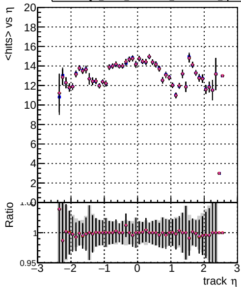
Legend: DQM mkFit XiMinusPU tetrain2-lowpt, DQM mkFit XiMinusPU NEWdefault specPless1-2-lowpt, DQM mkFit XiMinusPU NEWdefault specPless2-3-lowpt, DQM mkFit XiMinusPU NEWdefault specPless3-4-lowpt, DQM mkFit XiMinusPU NEWdefault specPless4-2-lowpt
