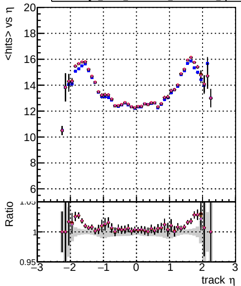
mean hits DQM mkFit XiMinusPU tetrain2-lowpt DQM mkFit XiMinusPU NEWdefault specPless1-2-lowpt DQM mkFit XiMinusPU NEWdefault specPless2-2-lowpt DQM mkFit XiMinusPU NEWdefault specPless3-2-lowpt DQM mkFit XiMinusPU NEWdefault specPless4-2-lowpt
