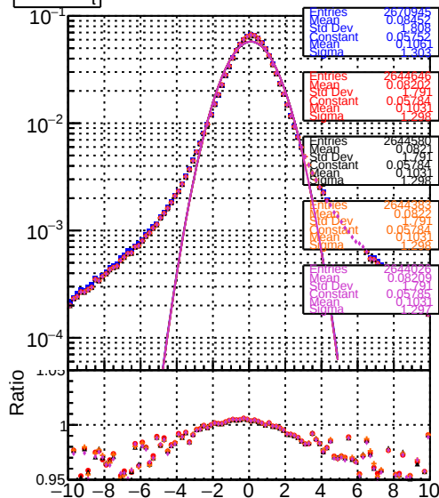
DOM mkFit YMinus PU retrain2 lowpt
