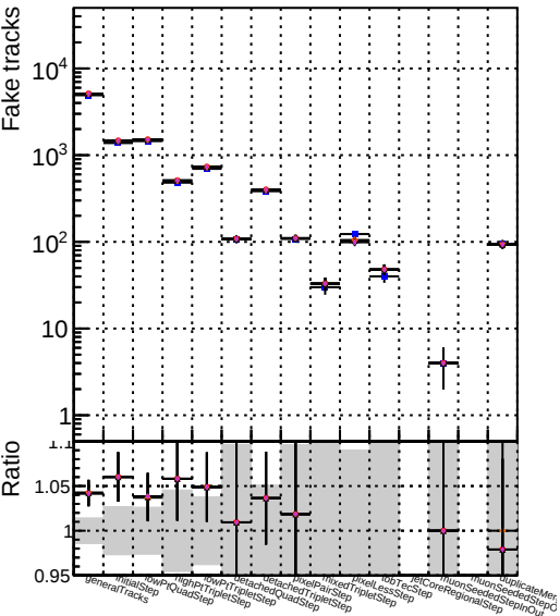
Number Symbol Model Configuration Method Configuration Method 1 DOM mkFit XiMinus PU NEWdefault 2 DOM mkFit XiMinus PU NEWdefault 3 DOM mkFit XiMinus PU NEWdefault
