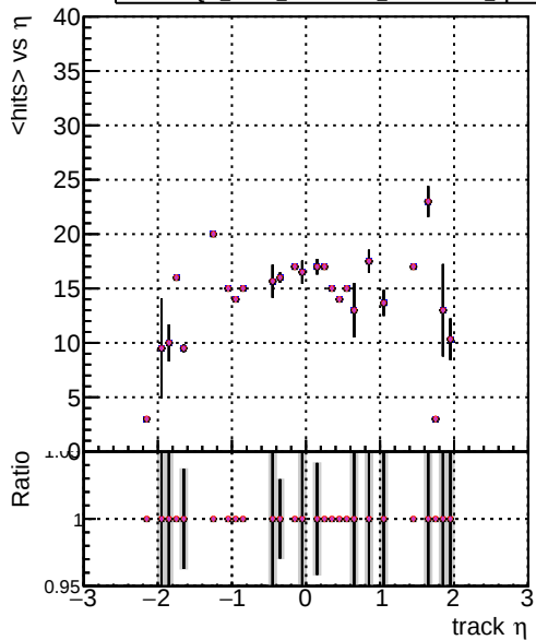
mean hit DQM mkFit XiMinusPU tetrax2-lowpt DQM mkFit XiMinusPU NEWdefault specPless1-2-lowpt DQM mkFit XiMinusPU NEWdefault specPless2-2-lowpt DQM mkFit XiMinusPU NEWdefault specPless3-2-lowpt DQM mkFit XiMinusPU NEWdefault specPless4-2-lowpt
