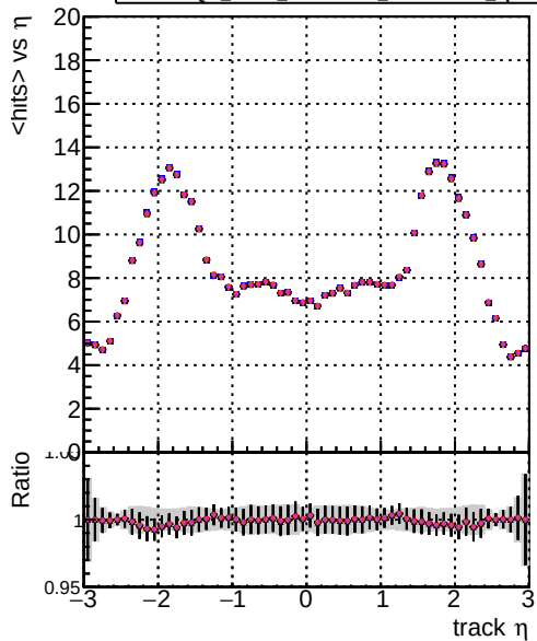
Legend: DQM mkFit XiMinusPU NEWdefault specPless1-2-lowpt, DQM mkFit XiMinusPU NEWdefault specPless2-2-lowpt, DQM mkFit XiMinusPU NEWdefault specPless3-2-lowpt, DQM mkFit XiMinusPU NEWdefault specPless4-2-lowpt
