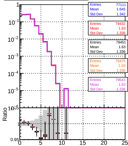
mean hits DQM mkFit XiMinusPU NEWdefault specPLess1-2-lowpt DQM mkFit XiMinusPU NEWdefault specPLess2-2-lowpt DQM mkFit XiMinusPU NEWdefault specPLess3-2-lowpt DQM mkFit XiMinusPU NEWdefault specPLess4-2-lowpt
