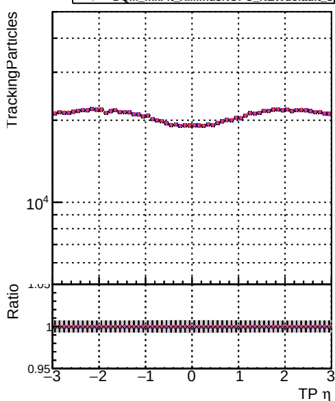
N of sin DOM mkFit XiMin DOM mkFit XiMin DOM mkFit XiMin 1 0.00 0.00 0.00 2 0.00 0.00 0.00 3 0.00 0.00 0.00 4 0.00 0.00 0.00 5 0.00 0.00 0.00 6 0.00 0.00 0.00 7 0.00 0.00 0.00 8 0.00 0.00 0.00 9 0.00 0.00 0.00 10 0.00 0.00 0.00 11 0.00 0.00 0.00 12 0.00 0.00 0.00 13 0.00 0.00 0.00 14 0.00 0.00 0.00 15 0.00 0.00 0.00 16 0.00 0.00 0.00 17 0.00 0.00 0.00 18 0.00 0.00 0.00 19 0.00 0.00 0.00 20 0.00 0.00 0.00 21 0.00 0.00 0.00 22 0.00 0.00 0.00 23 0.00 0.00 0.00 24 0.00 0.00 0.00 25 0.00 0.00 0.00 26 0.00 0.00 0.00 27 0.00 0.00 0.00 28 0.00 0.00 0.00 29 0.00 0.00 0.00 30 0.00 0.00 0.00 31 0.00 0.00 0.00 32 0.00 0.00 0.00 33 0.00 0.00 0.00 34 0.00 0.00 0.00 35 0.00 0.00 0.00 36 0.00 0.00 0.00 37 0.00 0.00 0.00 38 0.00 0.00 0.00 39 0.00 0.00 0.00 40 0.00 0.00 0.00 41 0.00 0.00 0.00 42 0.00 0.00 0.00 43 0.00 0.00 0.00 44 0.00 0.00 0.00 45 0.00 0.00 0.00 46 0.00 0.00 0.00 47 0.00 0.00 0.00 48 0.00 0.00 0.00 49 0.00 0.00 0.00 50 0.00 0.00 0.00 51 0.00 0.00 0.00 52 0.00 0.00 0.00 53 0.00 0.00 0.00 54 0.00 0.00 0.00 55 0.00 0.00 0.00 56 0.00 0.00 0.00 57 0.00 0.00 0.00 58 0.00 0.00 0.00 59 0.00 0.00 0.00 60 0.00 0.00 0.00 61 0.00 0.00 0.00 62 0.00 0.00 0.00 63 0.00 0.00 0.00 64 0.00 0.00 0.00 65 0.00 0.00 0.00 66 0.00 0.00 0.00 67 0.00 0.00 0.00 68 0.00 0.00 0.00 69 0.00 0.00 0.00 70 0.00 0.00 0.00 71 0.00 0.00 0.00 72 0.00 0.00 0.00 73 0.00 0.00 0.00 74 0.00 0.00 0.00 75 0.00 0.00 0.00 76 0.00 0.00 0.00 77 0.00 0.00 0.00 78 0.00 0.00 0.00 79 0.00 0.00 0.00 80 0.00 0.00 0.00 81 0.00 0.00 0.00 82 0.00 0.00 0.00 83 0.00 0.00 0.00 84 0.00 0.00 0.00 85 0.00 0.00 0.00 86 0.00 0.00 0.00 87 0.00 0.00 0.00 88 0.00 0.00 0.00 89 0.00 0.00 0.00 90 0.00 0.00 0.0
