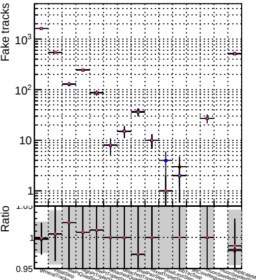
Number DQM mKFit XIMinusNOPU NEWdefault DQM mKFit XIMinusNOPU NEWdefault DQM mKFit XIMinusNOPU NEWdefault
