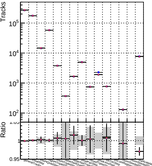
ROM - mkFit_XiMinusNOPU - newDefault5
