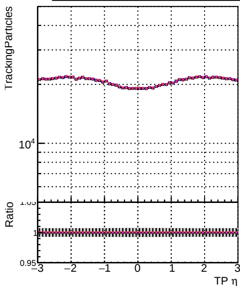
N of sin ↑ DQM mkFit XiMinusNOPU NEWdefault + DQM mkFit XiMinusNOPU NEWdefault ↓ DQM mkFit XiMinusNOPU NEWdefault
