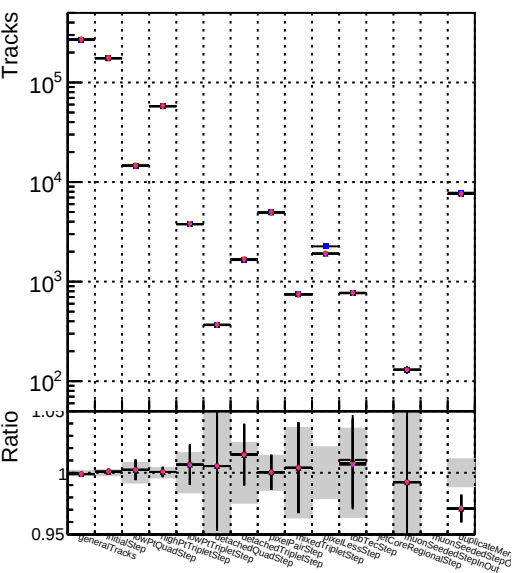
ROM - mkFit_XiMinusNOPU - newDefault5
