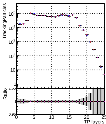
N of sim —●— DQM_mkFit_XiMinusNOP —●— DQM_mkFit_XiMinusNOP
