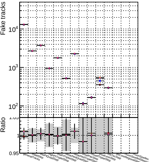
Number ★ DOM mkFit XiMinusNOPIU NEWdefault ✱ DOM mkFit XiMinusNOPIU NEWdefault — DOM mkFit XiMinusNOPIU NEWdefault
