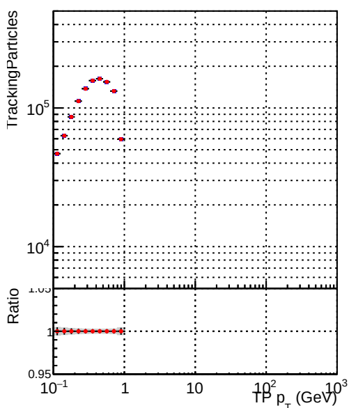
—•— DQM_mkFit_XiMinusNOPU_newDefault5 —•— DQM_mkFit_XiMinusNOPUold-lowpt
