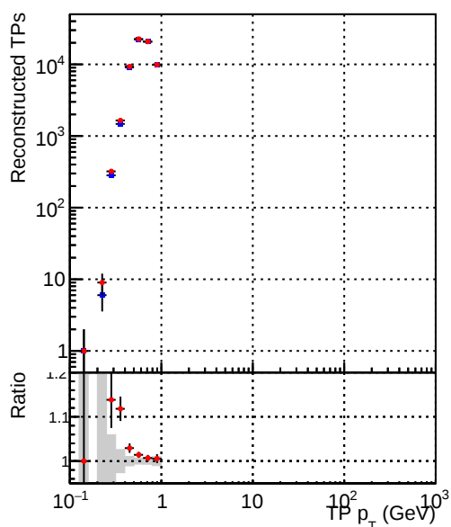
■ DQM_mkFit_XiMinusNOPU_newDefault5 ■ DQM_mkFit_XiMinusNOPUold-lowpt
