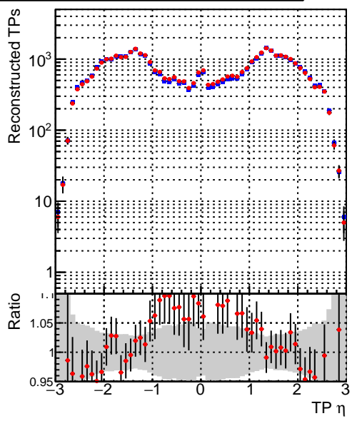
Legend: DQM_mkFit_XiMinusNOPU_newDefault5 (blue squares), DQM_mkFit_XiMinusNOPUold-lowpt (red circles)
