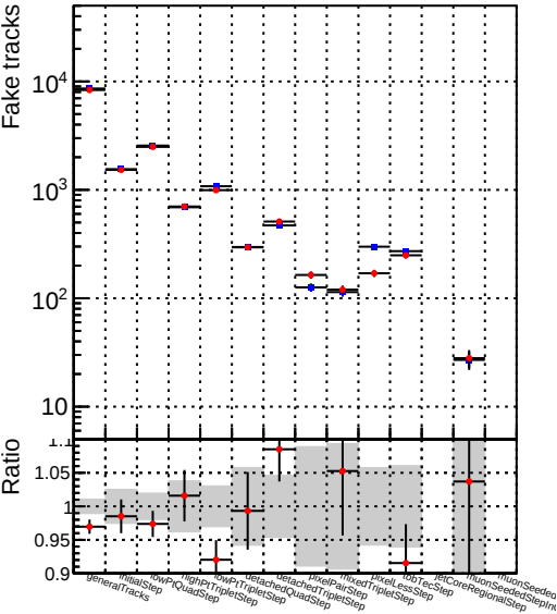
Number —●— DQM_mkFit XiMinusNOPUold-lowpt
