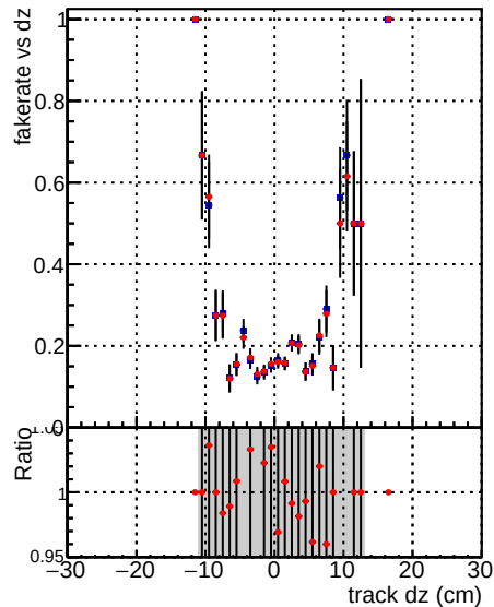
—●— DQM_mkFit_XiMinusNOPU_newDefault5 —●— DQM_mkFit_XiMinusNOPUold-lowpnt
