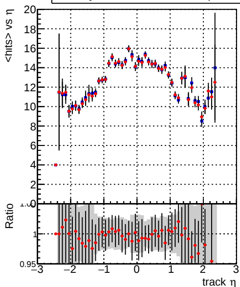
— DQM_mkFit_XiMinusNOPU_newDefault5 — DQM_mkFit_XiMinusNOPUold-lowpt
