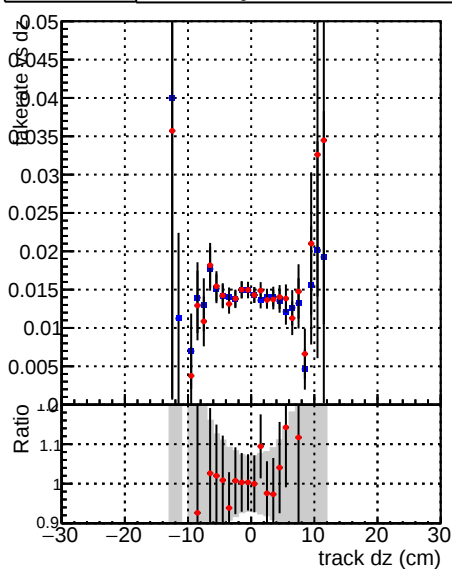
— DQM_mkFit_XiMinusNOPU_newDefault5 — DQM_mkFit_XiMinusNOPUold-lowpt
