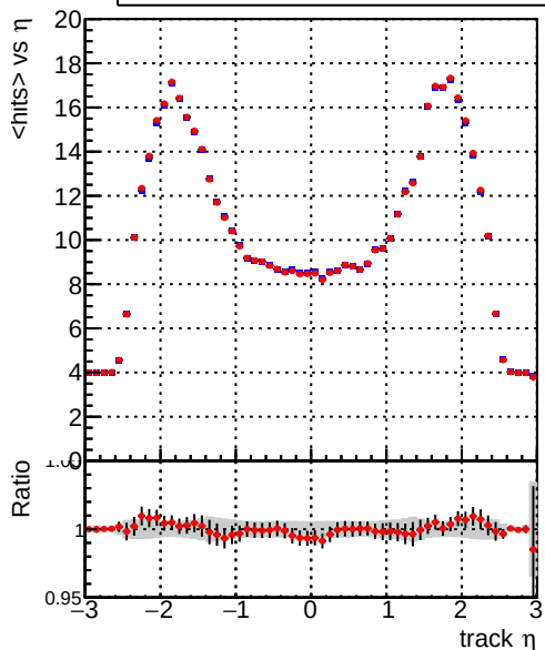
mean hit — DQM_mkFit_XiMinusNOPU_newDefault5 — DQM_mkFit_XiMinusNOPUold-lowpt
