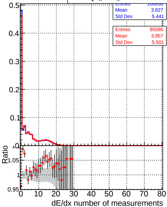
DQM_mkFit_XiMinusNOPU_newDefault5 DQM_mkFit_XiMinusNOPUold-lowpt
