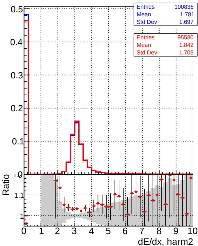
DQM_mkFit_XiMinusNOPU_newDefault5 DQM_mkFit_XiMinusNOPUold-lowpt
