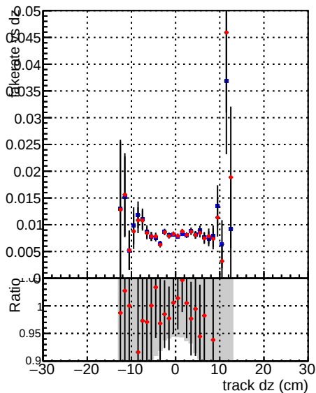
— DQM_mkFit_XiMinusNOPU_newDefault5 — DQM_mkFit_XiMinusNOPUold-lowp
