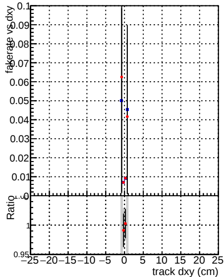
— DQM_mkFit_XiMinusNOPU_newDefault5 — DQM_mkFit_XiMinusNOPUold-lowp
