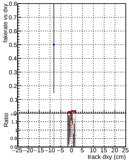
—●— DQM_mkFit_XiMinusNOPU_newDefault5 —●— DQM_mkFit_XiMinusNOPUold-lowpt
