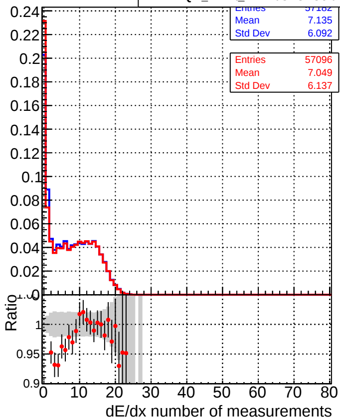
—■— DQM_mkFit_XiMinusNOPU_newDefault5 —●— DQM_mkFit_XiMinusNOPUold-lowpt
