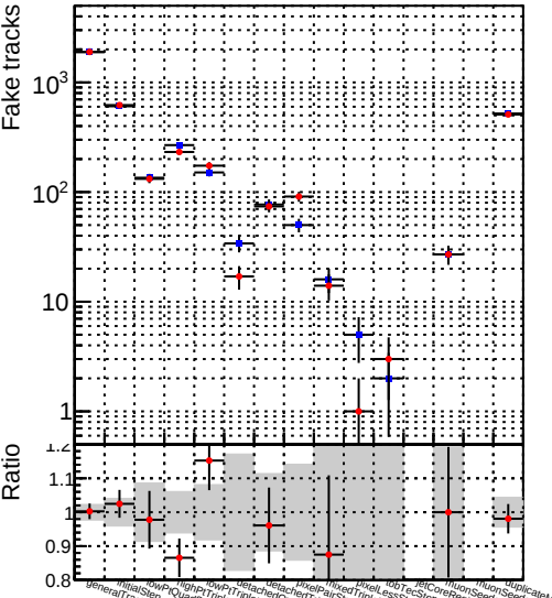
Number —●— DQM_mkFit_XiMinusNOPUold-lowpt
