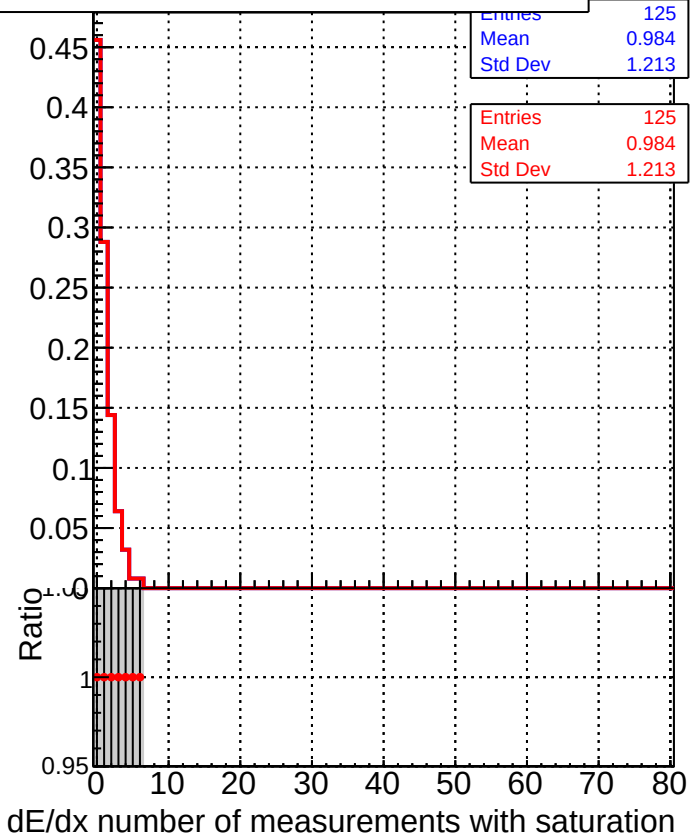
DQM_mkFit_XiMinusNOPU_newDefault5 DQM_mkFit_XiMinusNOPUold-lowpt
