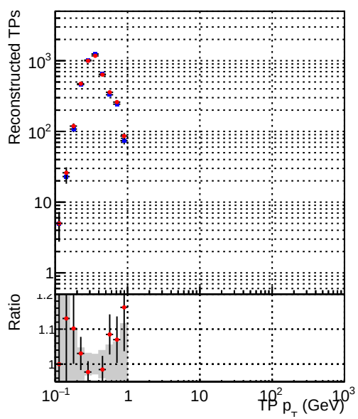
—•— DQM_mkFit_XiMinusNOPU_newDefault5 —•— DQM_mkFit_XiMinusNOPUold-lowpt
