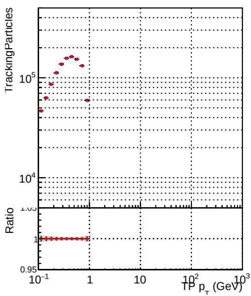
—•— DQM_mkFit_XiMinusNOPU_newDefault5 —•— DQM_mkFit_XiMinusNOPUold-lowpt
