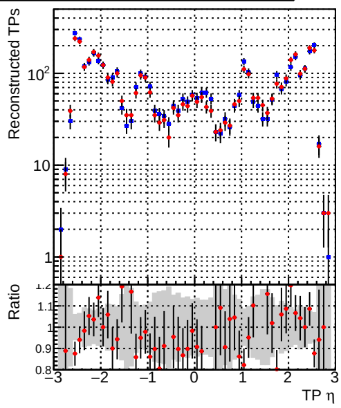
—•— DQM_mkFit_XiMinusNOPU_newDefault5 —•— DQM_mkFit_XiMinusNOPUold-lowpt
