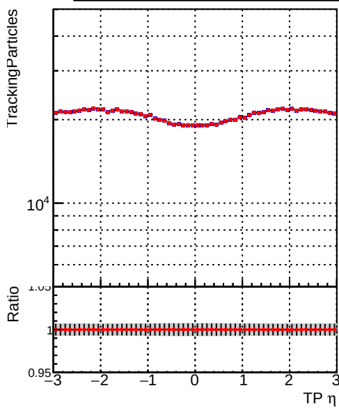
—•— DQM_mkFit_XiMinusNOPU_newDefault5 —•— DQM_mkFit_XiMinusNOPUold-lowpt
