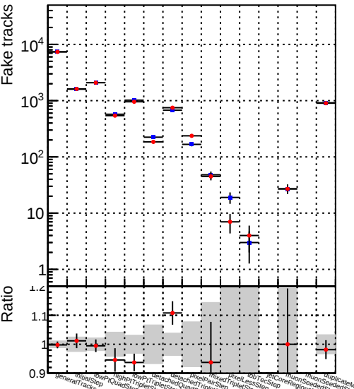
Number —●— DQM_mkFit_XiMinusNOPUold-lowpt
