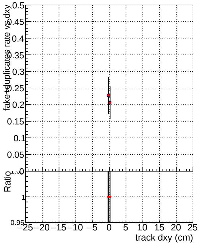
DQM_mkFit_XiMinusNOPU_newDefault5 DQM_mkFit_XiMinusNOPUold-lowpt
