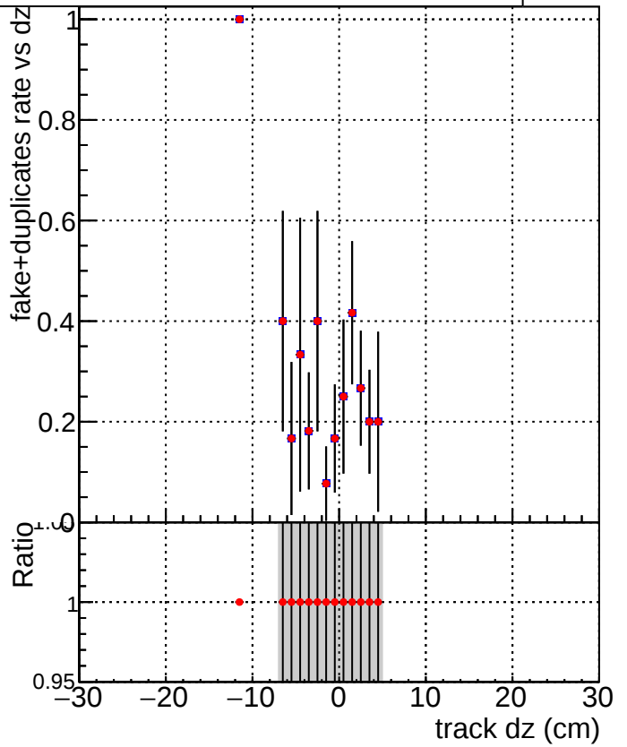
DQM_mkFit_XiMinusNOPU_newDefault5 DQM_mkFit_XiMinusNOPUold-lowpt
